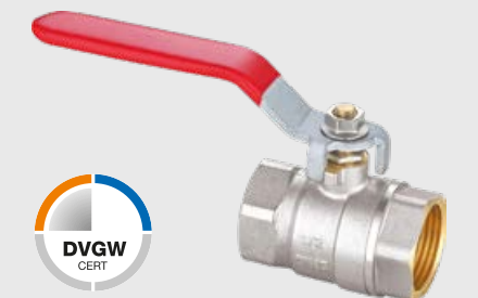
Kugelhahn IG x IG DVGW konform. Kugelhähne sind Trinkwasserneutral (DW-6102CU0310).
